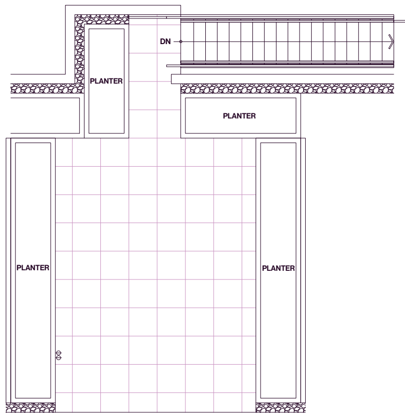
ROOFDECK
