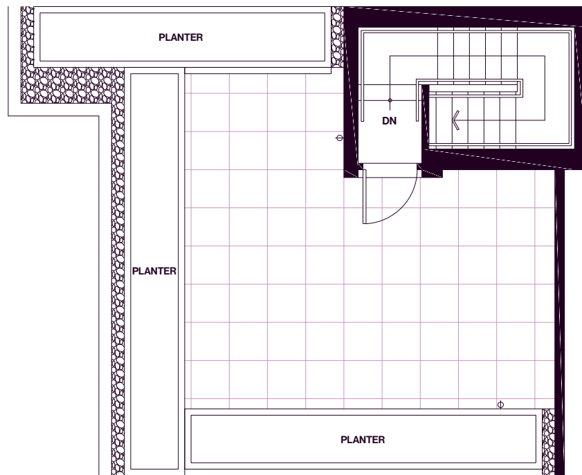
ROOFDECK
